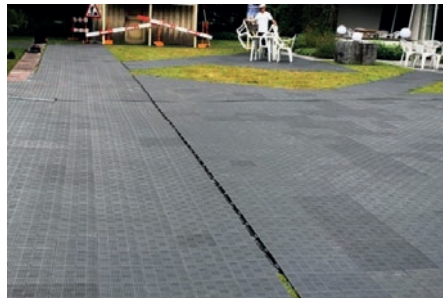
Bild 4: Richtig! Dehnungsfuge gleicht Wärmeausdehnung aus
